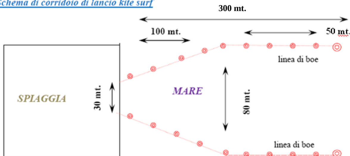
Schema di corridoio di lancio kite surf
