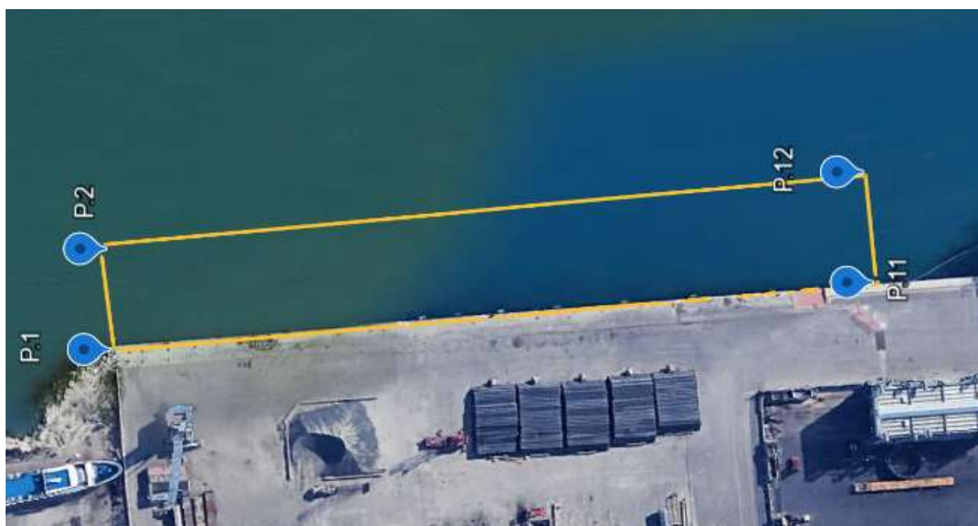
ALL. 1 - PLANIMETRIA GENERALE DELLO SPECCHIO ACQUEO INTERESSATO DALLE ATTIVITA' DI INFISSIONE DI COMBI WALL IN PROSSIMITA' DELLA BANCHINA DI RIVA
